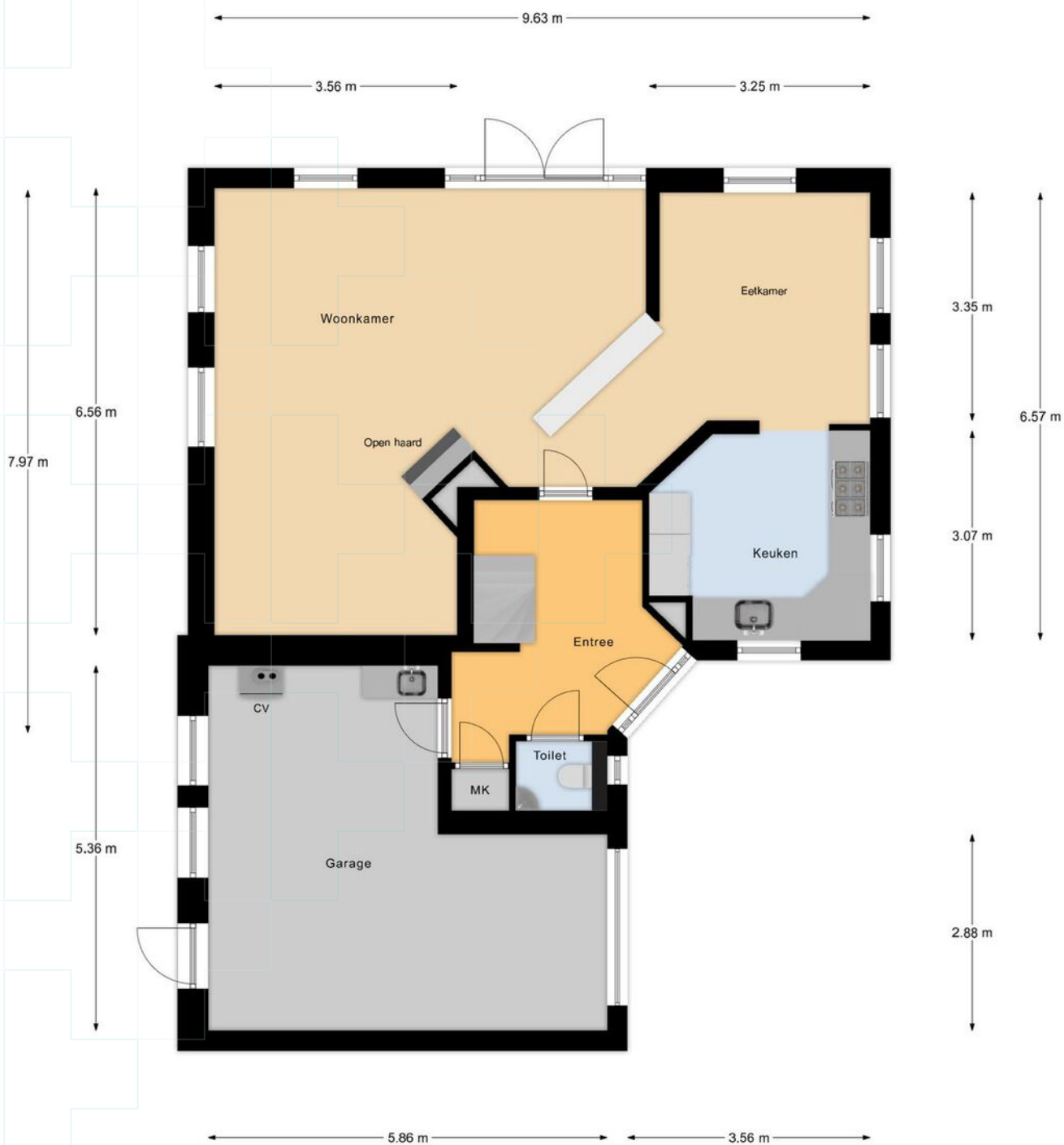
Begane Grond
